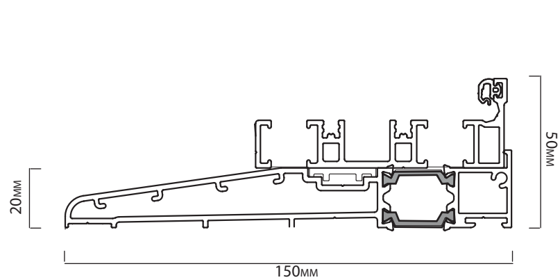
CILL
